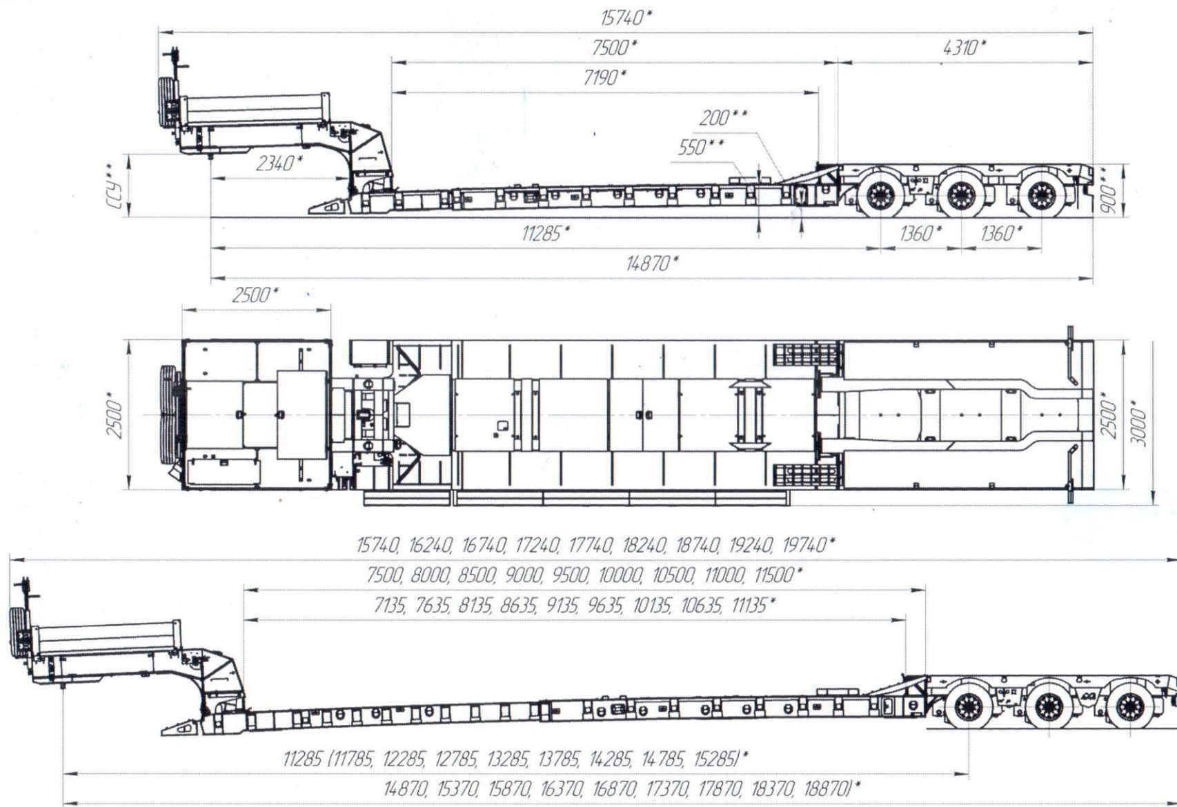
Рис.1. Полуприцеп автомобильный 994293 00.00.000 ПС
